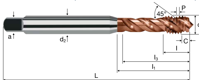
EC10550 / DIN 371 (EC 10551 / DIN 376 non mostrato)
