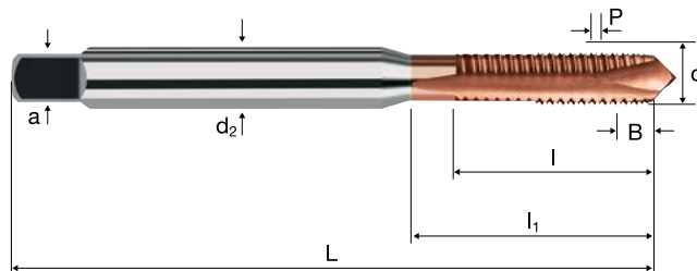
EC10540 / DIN 371 (EC 10541 / DIN 376 non mostrato)
