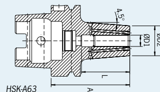
HSK-A63
