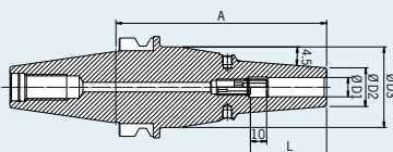
BT40
